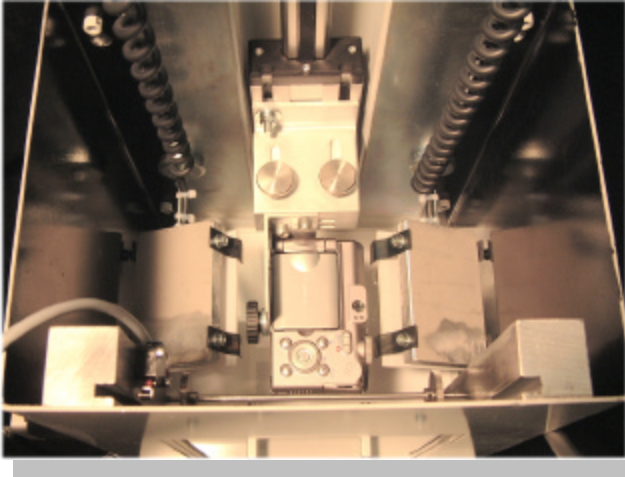
Motorisierte Kamerahalterung [ Bildfeld 20 – 200 mm ]
